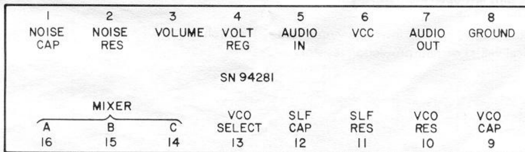
IC PINOUT
